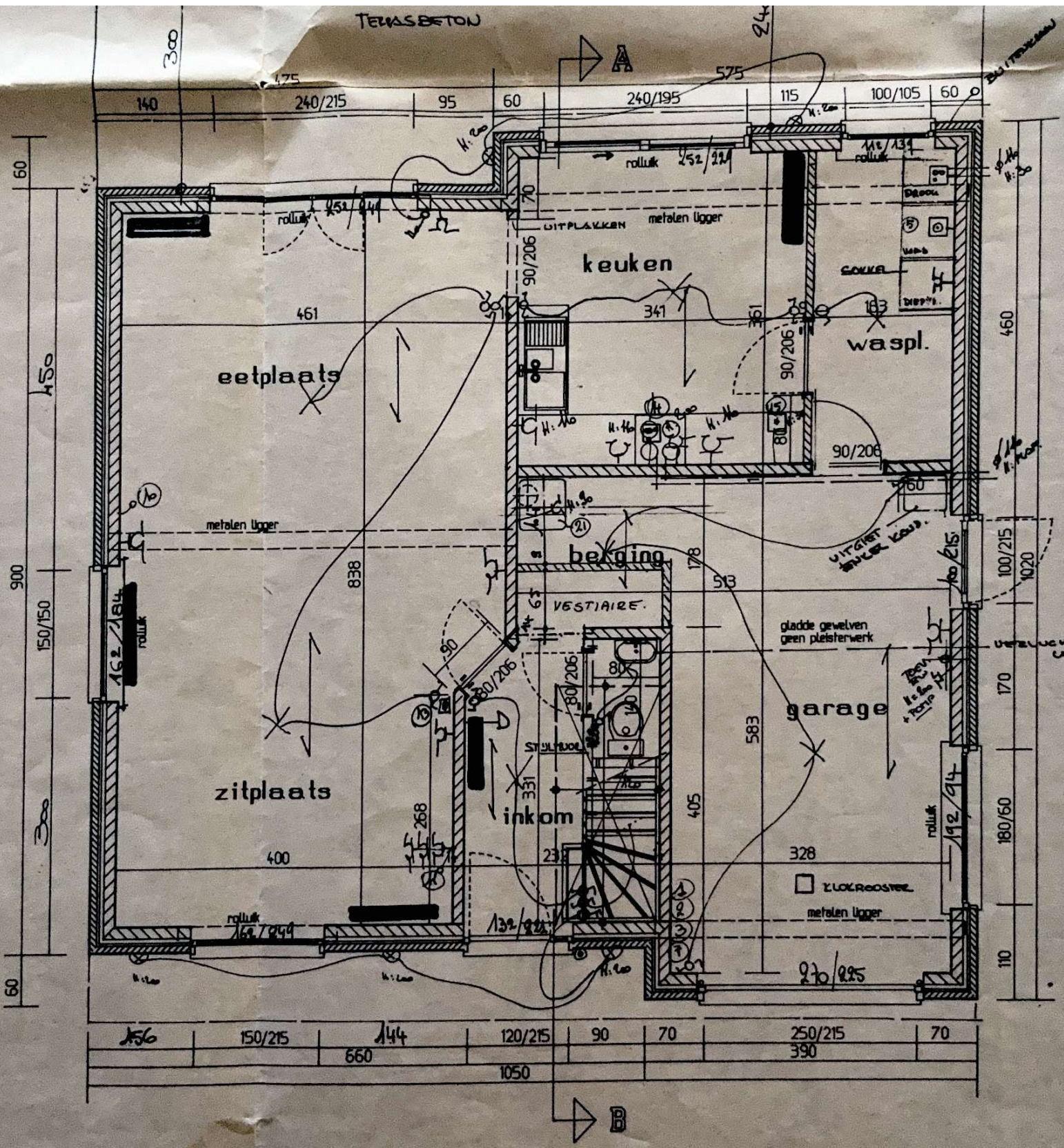
GRONDPLAN
